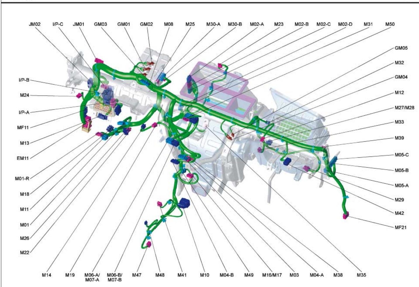
主线束(1)
